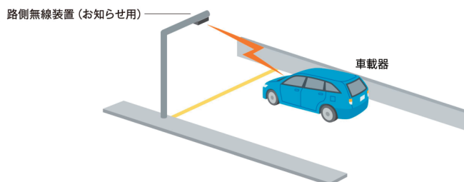
ETCカード未挿入お知らせアンテナの機器配置例
